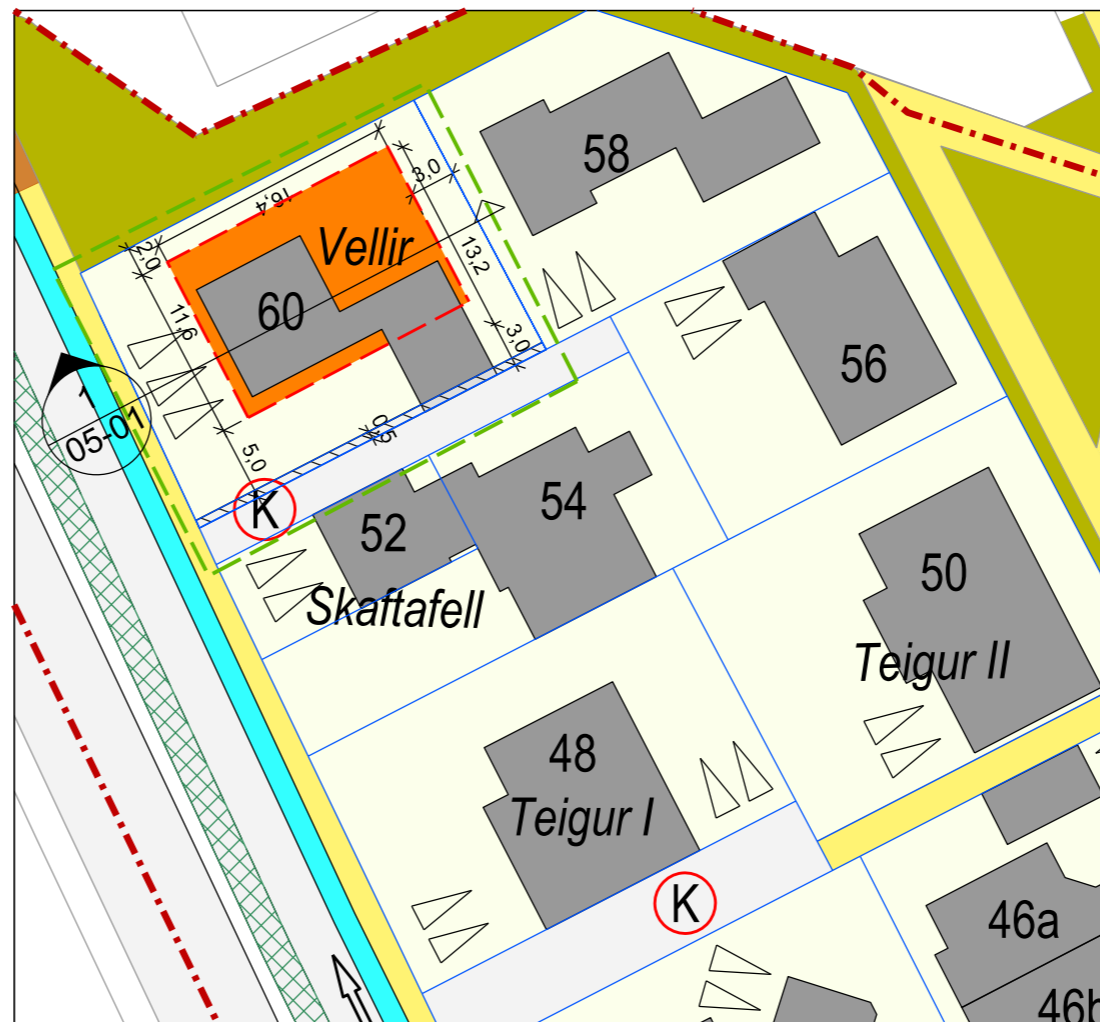
BREYTT DEILISKIPULAG. KVARDI 1:500
