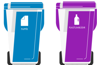
Mars
